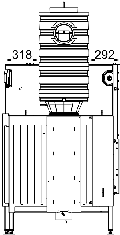
~1:20 sortie arrière, adaptateur excentrique
