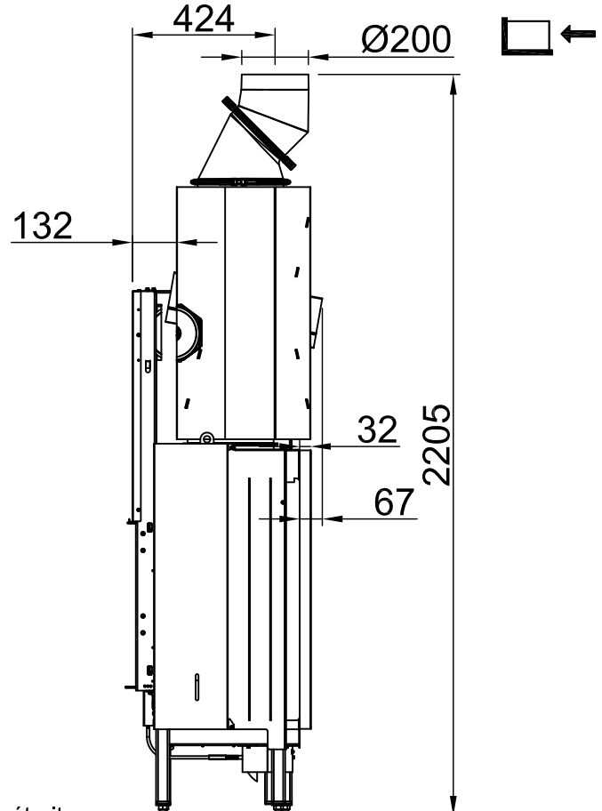
Thermobox, étroite
