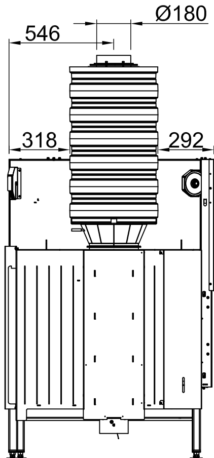
~1:20 sortie haut, adaptateur excentrique
