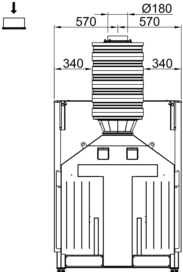
~1:20 Scarico superiore, Adattatore escentrico
