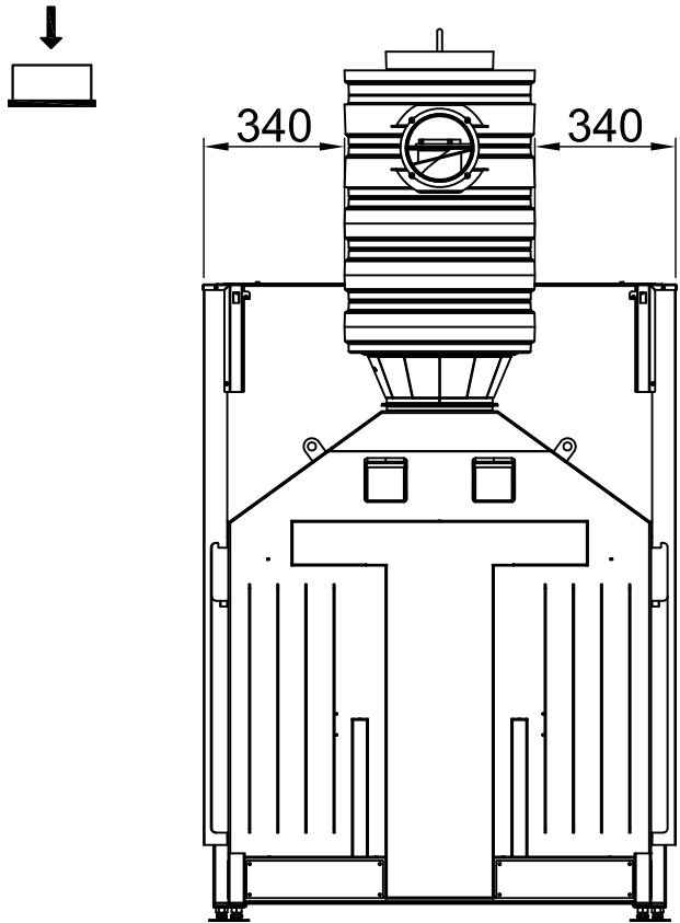
~1:20 Scarico posteriore, Adattatore escentrico
