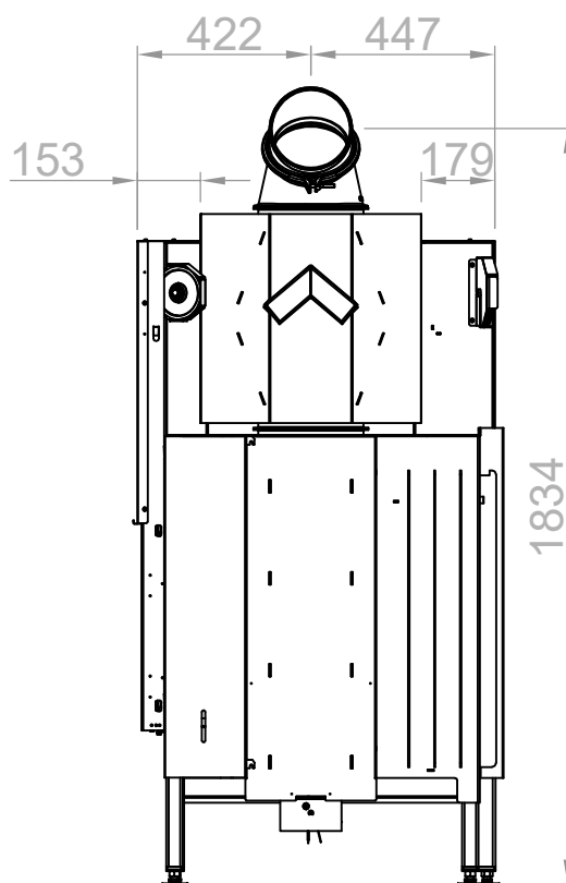
Thermobox, breit
