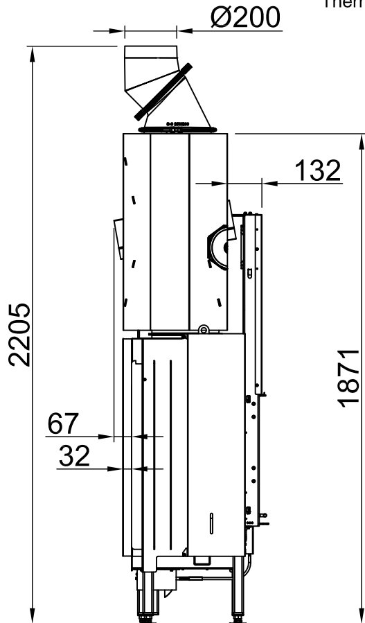
Thermobox, étroite
