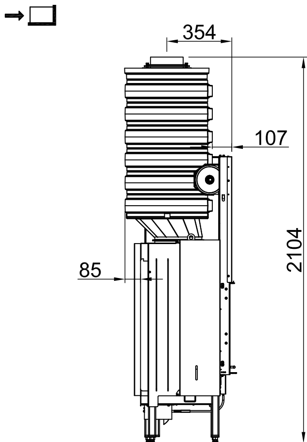
~1:20 sortie haut, adaptateur excentrique
