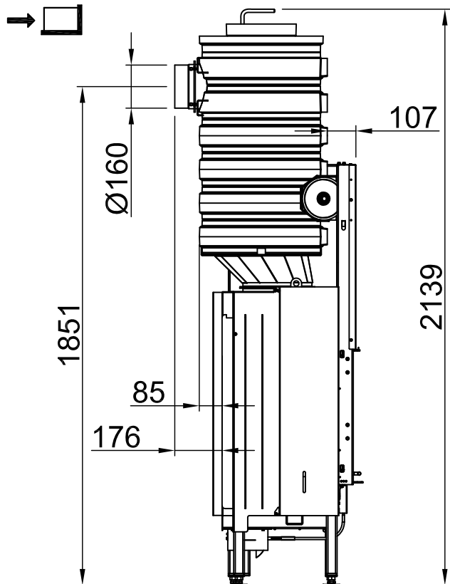
~1:20 sortie arrière, adaptateur excentrique
