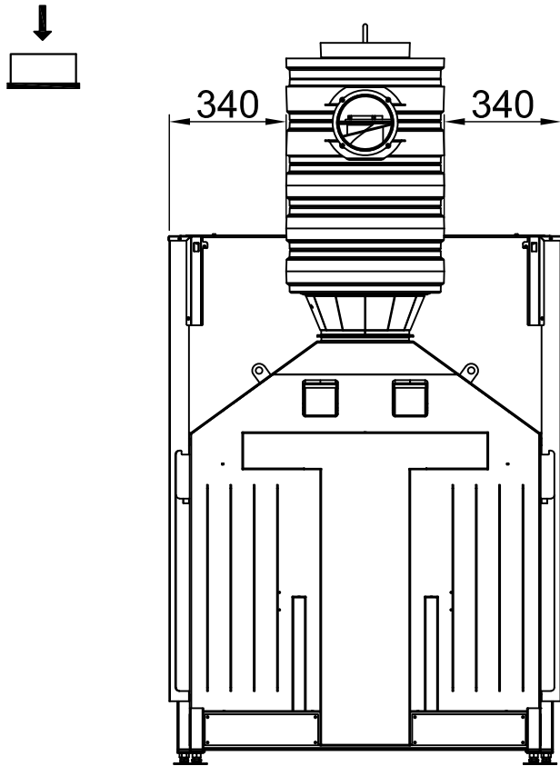
~1:20 salida, trasera, adaptador excéntrico
