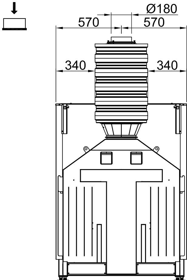
~1:20 salida, arriba, adaptador excéntrico
